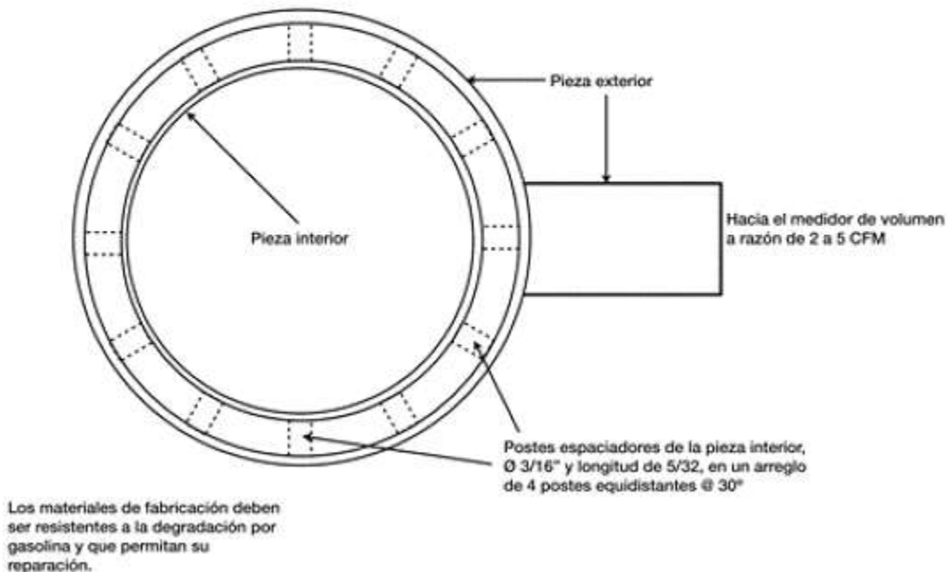
Figura 1. Captador de vapores, vista de planta.
